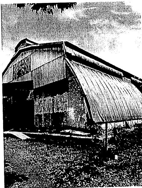
Figura 11: A edificação apresenta uma estrutura de shed semicircular, onde o fechamento lateral e a cobertura são contínuos. A porção inferior da parede é construída em alvenaria de vedação, que recebeu acabamento de reboco e pintura. A porção superior curva é totalmente revestida externamente com chapas metálicas corrugadas (telhas de zinco), que definem o formato do arco.
